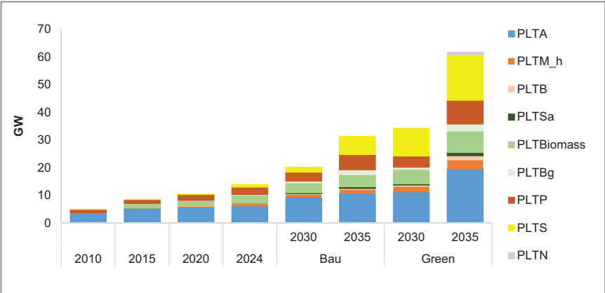
Gambar 3.5 Kapastias Pembangkit Listrik EBT per Jenis Pembangkit
